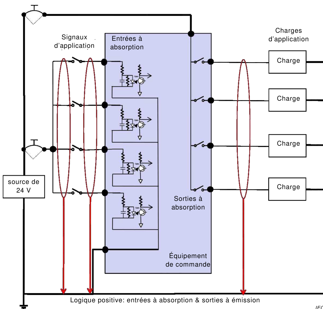
Figure F.2 – Logique positive avec défauts
