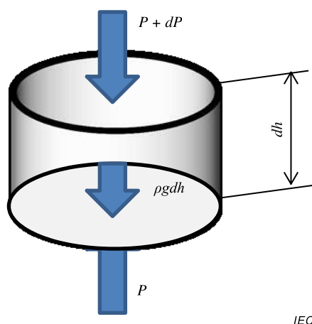
Figure A.1 – Petit élément atmosphérique
