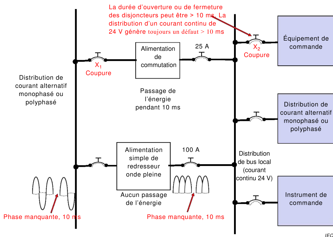
Figure E.1 – Distribution de courant continu aux équipements de commande et défauts
