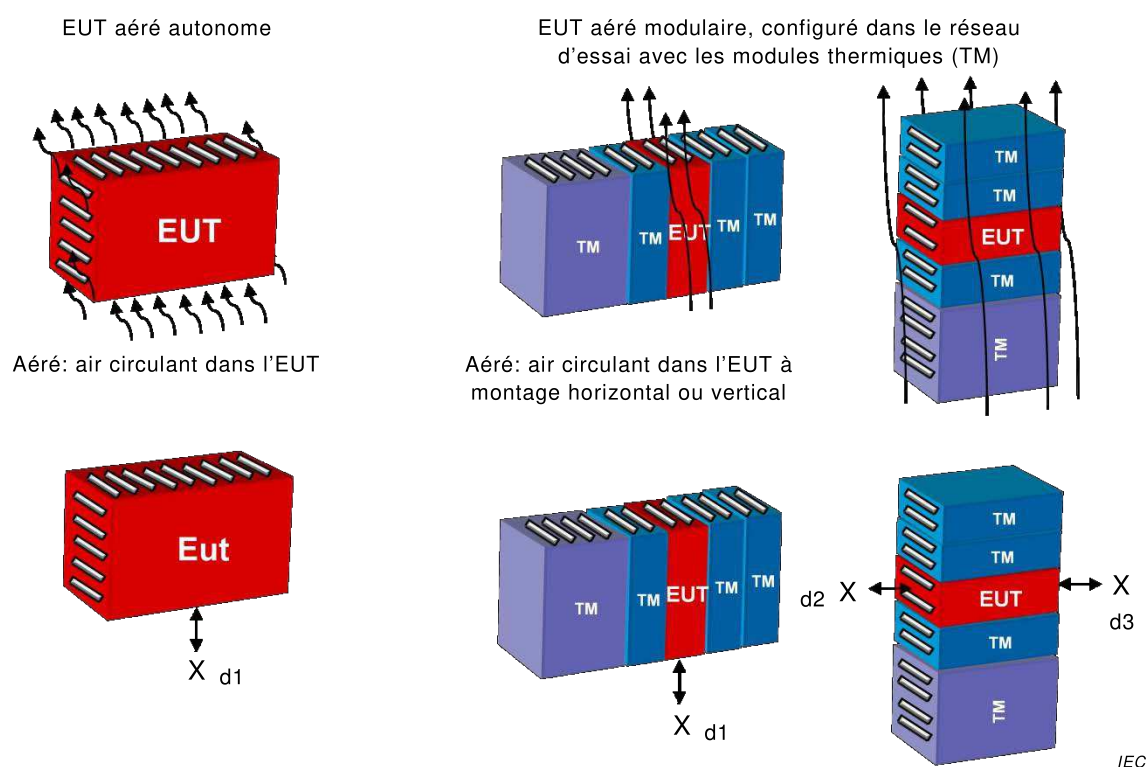
Figure 4 – Équipement aéré
